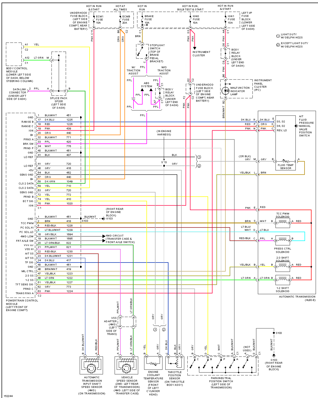
Fig. 84: 6.0L VIN U, A/T Circuit, 4L80-E
