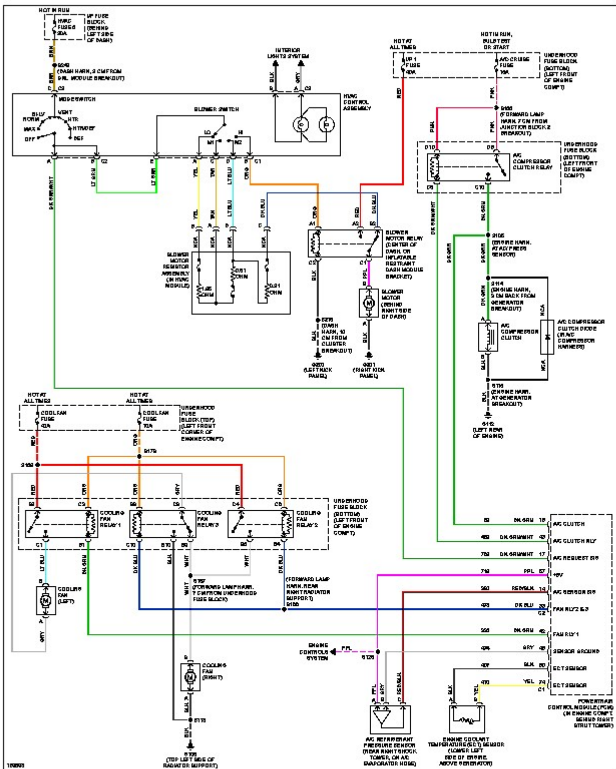
Fig. 4: 5.7L VIN G, Manual A/C Circuit
