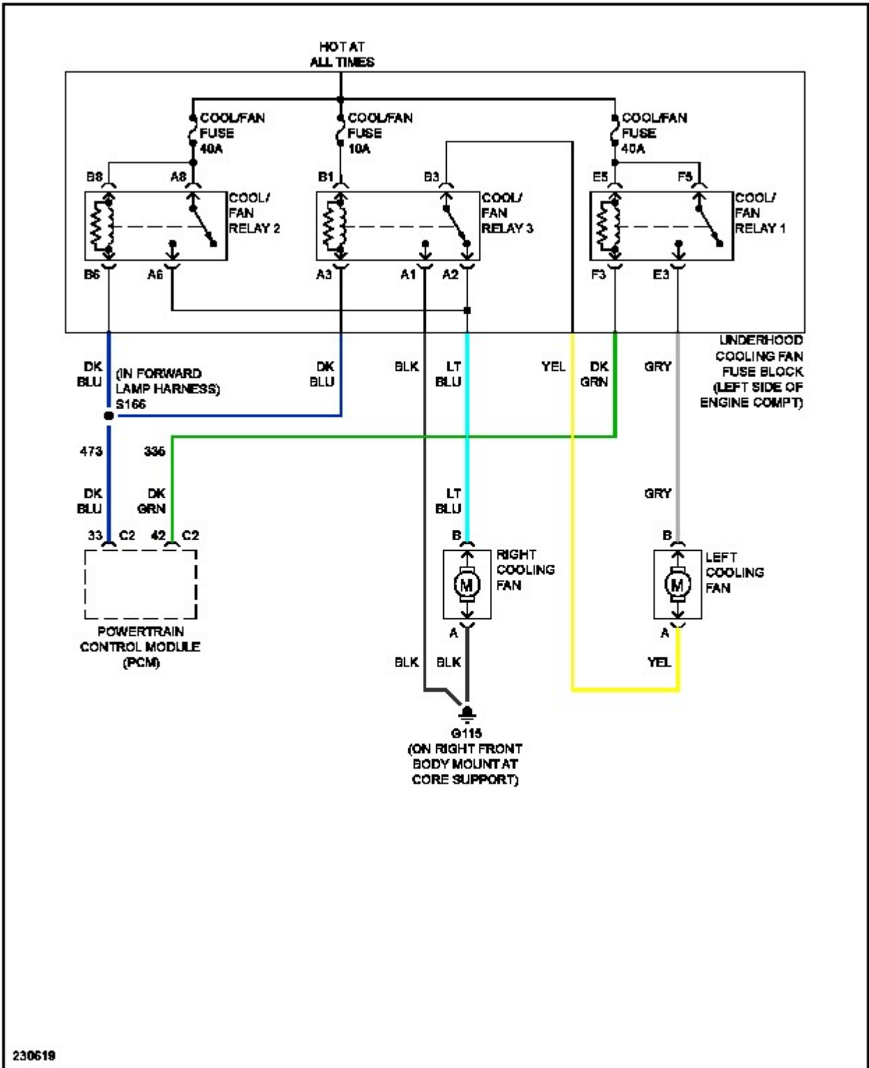
Fig. 22: Cooling Fan Circuit
