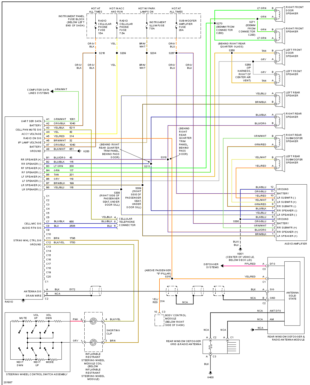
Fig. 37: Radio Circuit
