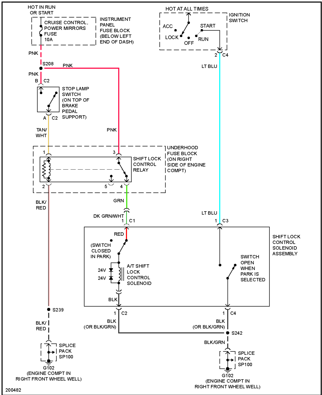
Fig. 38: Shift Interlock Circuit
